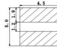
Land patterns 贴装尺寸(mm)
